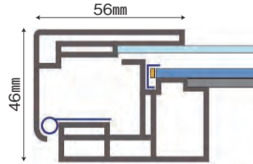
アルミフレーム断面略図
